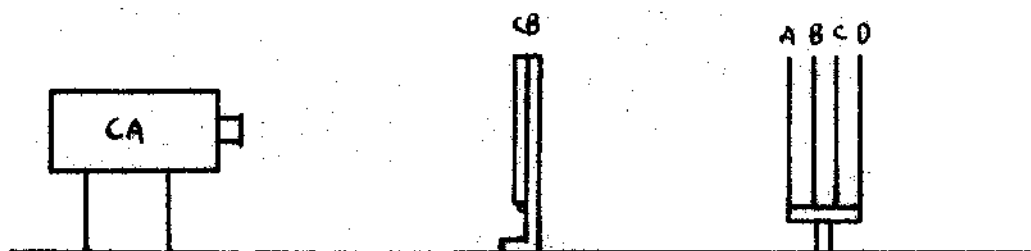
Fig. 3. Schema Ub Iwerks - A, B, C: vetro (o cartone) - D, fondo - CA: apparecchio da presa - CB: sostegno per la scena (celluloidi).
