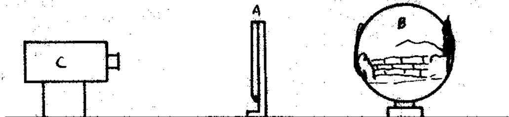
Fig. 2. Schema Fleischer - A, sostegno per la scena su celluloidi (movimento) - B, 'Travelling' plastico - C, apparecchio da presa.
